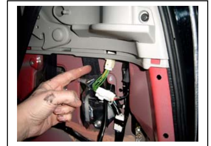
obere Steckverbindung lösen, Kabelbaum dazwischen anschließen
