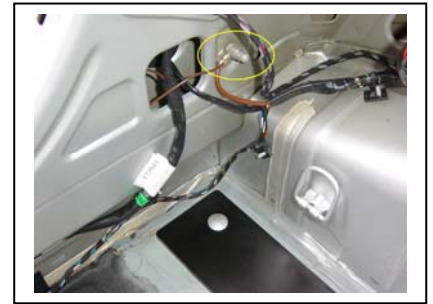
Massekabel festschrauben
